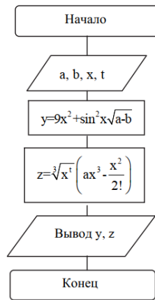
Рисунок 11 – Алгоритм решения задачи
