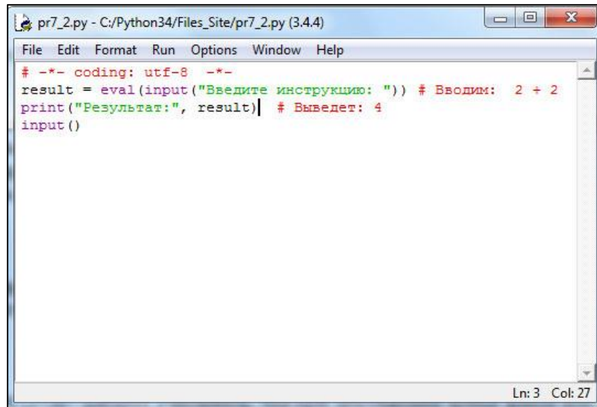
Рисунок 3 – Использование функции eval ()
