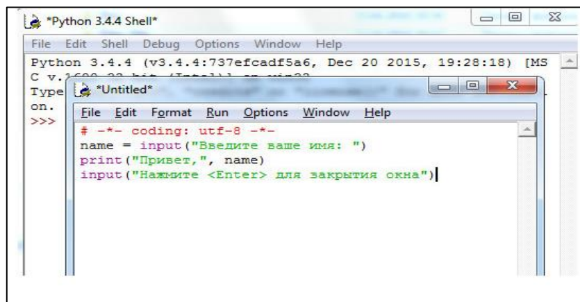
Рисунок 2 – Пример использования функции input ()
