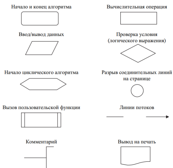
Рисунок 1 – Функциональные блоки при отрисовке блок-схем
